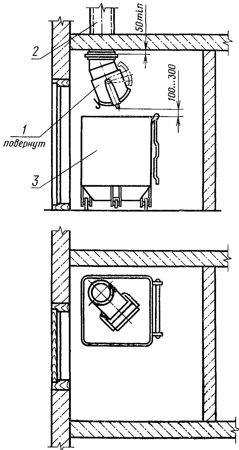
1—шибер; 2—ствол мусоропровода; 3—контейнер Черт. 2
