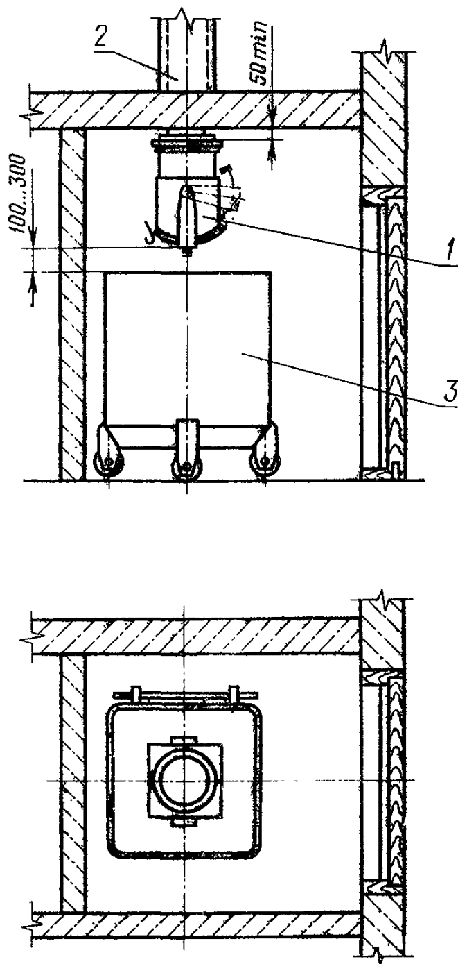
1—шибер; 2—ствол мусоропровода; 3—контейнер Черт. 1
