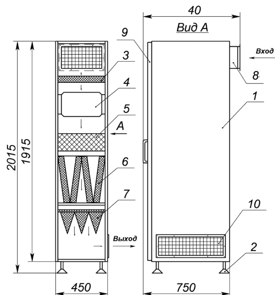
1 - корпус блока; 2 - опоры; 3 - фильтр гофрированный ФЯГ; 4 - вентилятор; 5 - фильтр складчатый ФЯС; 6 - ячейки угольного фильтра ЯУФ2; 7 - фильтр карманный с ионообменным материалом; 8 - входной патрубок с решеткой; 9 - съемная дверца; 10 - выходная решетка.
