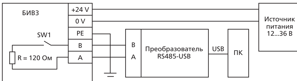
Схема подключения БИВЗ к персональному компьютеру
