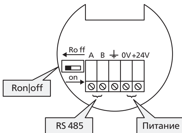
Назначение контактов клеммного соединителя БИВЗ
