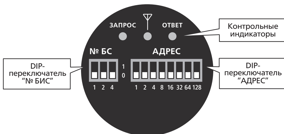
РИСУНОК 5 Табло блока БИВ2
