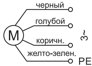
Схема подключения №4
