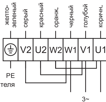
Схема подключения №6
