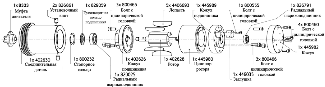
Рисунок 2.17. Детализировка пневматического двигателя JP-AIR 1.
