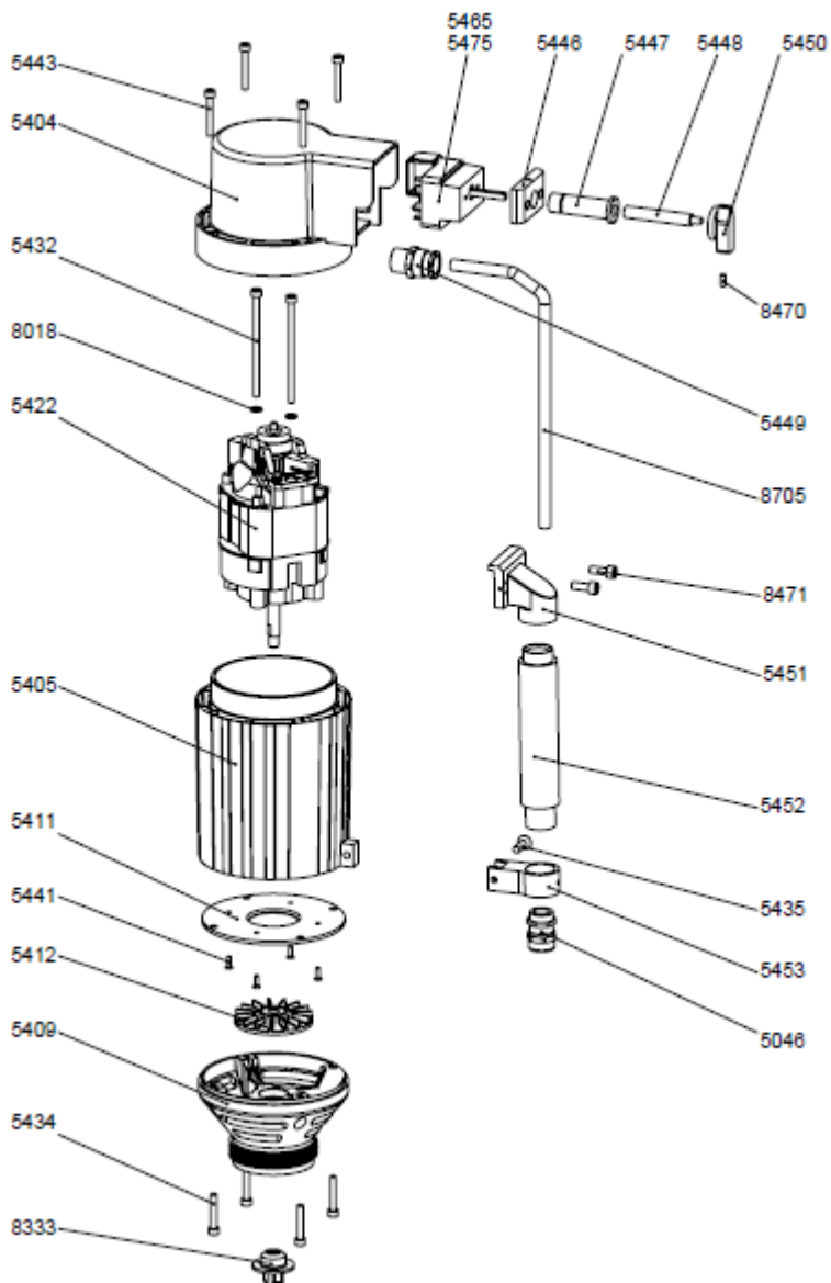
Рисунок 2.16. Детализировка электродвигателя JP-480.
