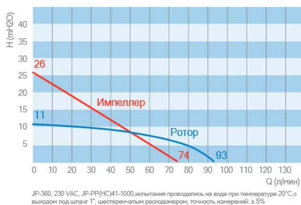
Рисунок 1.7. График JP-360.
