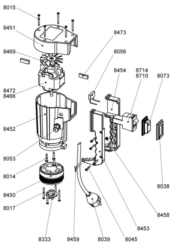
Рисунок 2.5. Деталировка электродвигателя JP-120 и 140 (выпуск до 2019 г., арт. 1140 XXXX).
