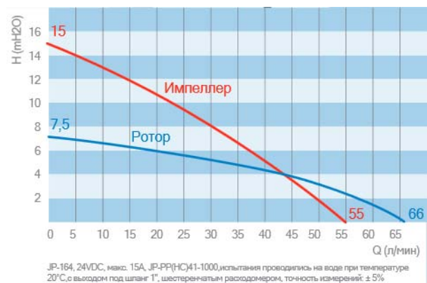
Рисунок 1.4. График JP-164.
