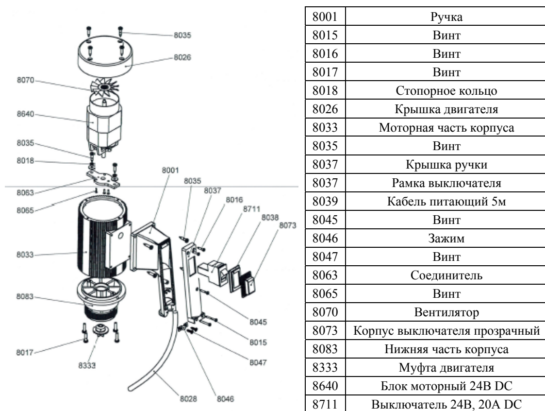
Рисунок 2.7. Детализовка электродвигателя JP-164.
