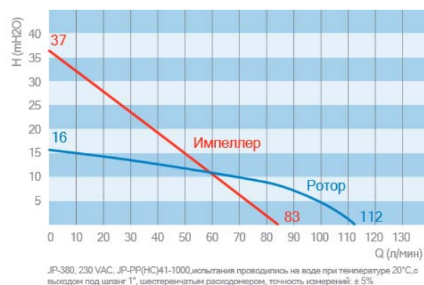
Рисунок 1.8. График JP-380.
