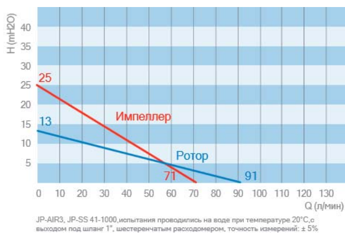
Рисунок 1.15. График JP-AIR 3.
