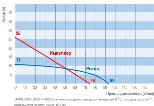
Рисунок 1.11. График JP-460.
