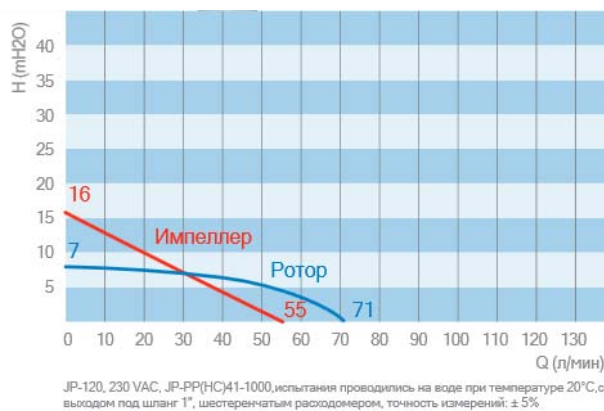
Рисунок 1.1. График JP-120.
