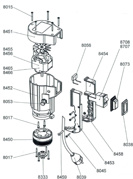
Рисунок 2.5. Деталировка электродвигателя JP-120 и 140 (выпуск до 2019 г., арт. 1140 XXXX).
