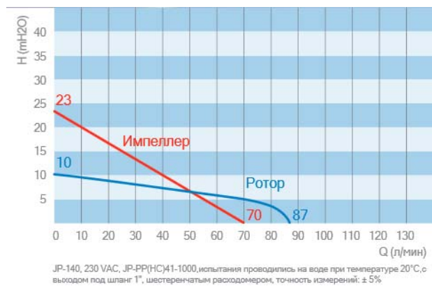
Рисунок 1.2. График JP-140.
