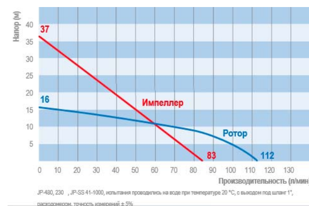
Рисунок 1.12. График JP-480.
