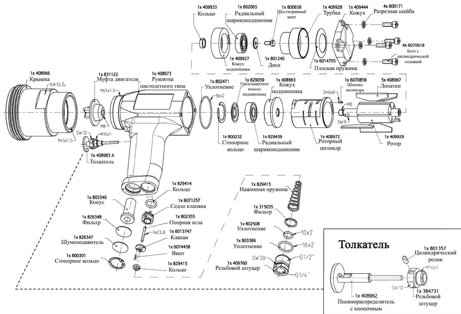
Рисунок 2.18. Деталировка пневматического двигателя JP-AIR 2.
