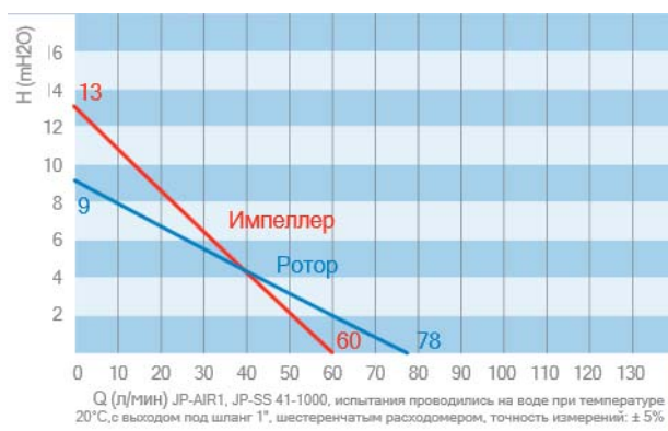
Рисунок 1.13. График JP-AIR 1.
