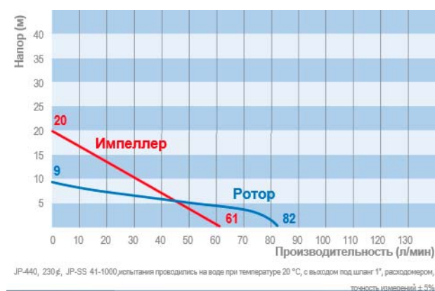
Рисунок 1.10. График JP-440.
