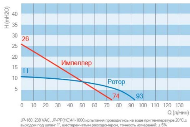
Рисунок 1.5. График JP-180.
