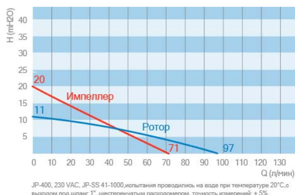
Рисунок 1.9. График JP-400.
