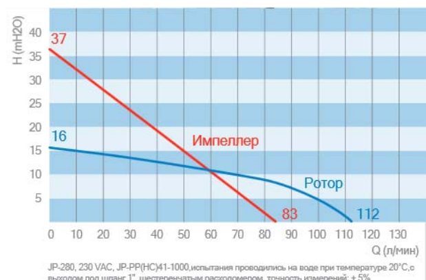
Рисунок 1.6. График JP-280.
