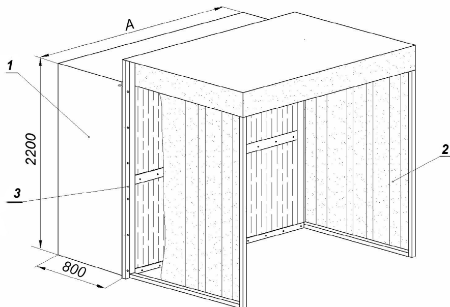
Рис.1. Схема покрасочной камеры
