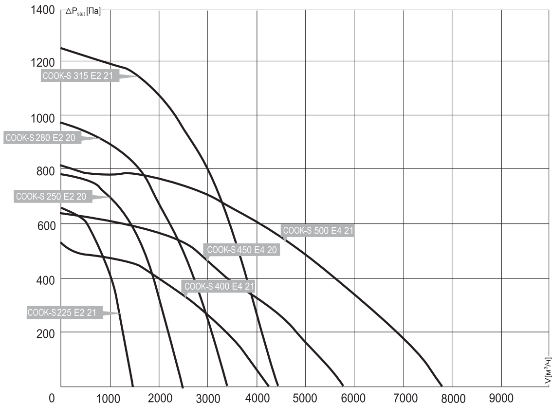
ГРАФИК ПАДЕНИЯ ДАВЛЕНИЯ COOK-S
