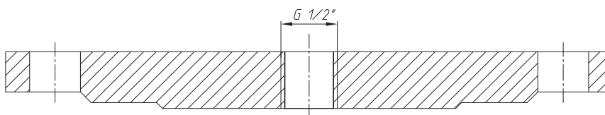
РИСУНОК 5. Крышка фланца с резьбой G \frac{1}{2} "
