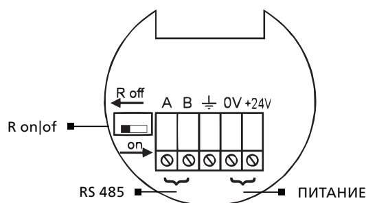
РИСУНОК 29. Назначение контактов клеммного соединителя уровнемеров ВЕКТОРХ-XXXU Вн, ВЕКТОРХХХХU-ДТ-Вн
