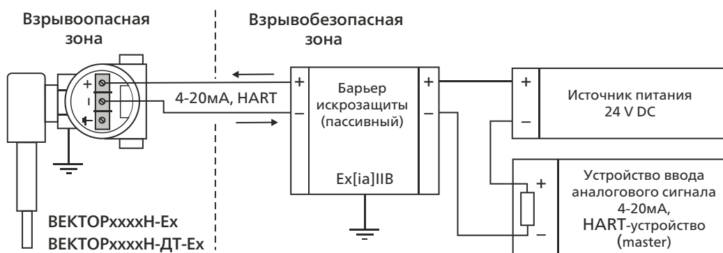
РИСУНОК 27. Схема подключения уровнемеров ВЕКТОРXXXXН-Ex, ВЕКТОРXXXXН-ДТ-Ex без гальванической развязки искробезопасных цепей.
