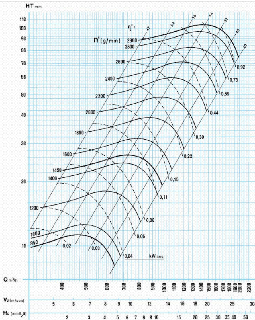
Рис. 3. Функциональная диаграмма вентиляторов VSB 20 (Величины давлений H_d и H_t приведены в миллиметрах водяного столба, 1 мм H_2O \sim 10 Pa)
