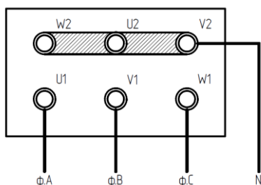
Подключение по схеме «звезда»
