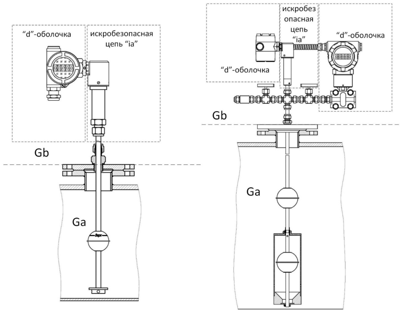
Рисунок 6. СХЕМАТИЧНОЕ РАСПОЛОЖЕНИЕ УРОВНЕМЕРА В ЗОНАХ Ga И Gb
