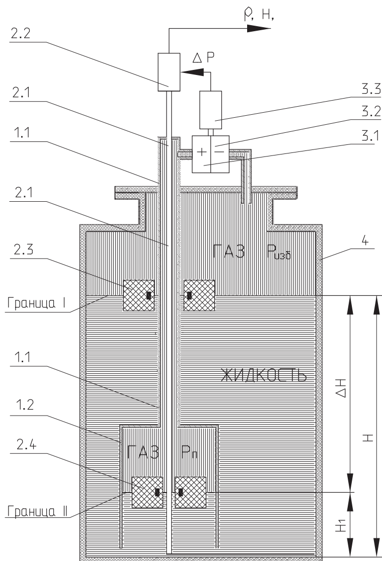
РИСУНОК 5. ПРИНЦИПИАЛЬНОЕ УСТРОЙСТВО УРОВНЕМЕРА ВЕКТОРXXXXН(У)-ДПТ
