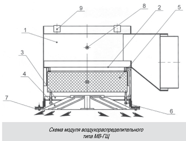
Рис. 6 Схема модуля MB с воздухораспределительной решеткой в четыре стороны
