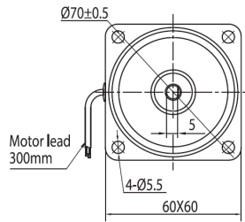
● ЭЛЕКТРОДВИГАТЕЛЬ (Вес: 1,1кг)
