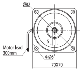
● ЭЛЕКТРОДВИГАТЕЛЬ (Вес: 1,45кг)
