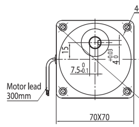
● МОТОР-РЕДУКТОР (Вес: 1,6кг)
