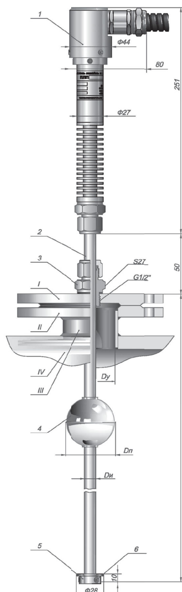
РИСУНОК В.6 Габаритно-установочный чертеж ПЛП1xxx-У-T2
